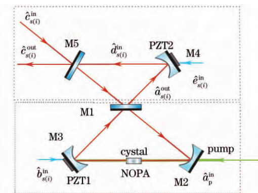
图 1 相干反馈控制 NOPA 系统
