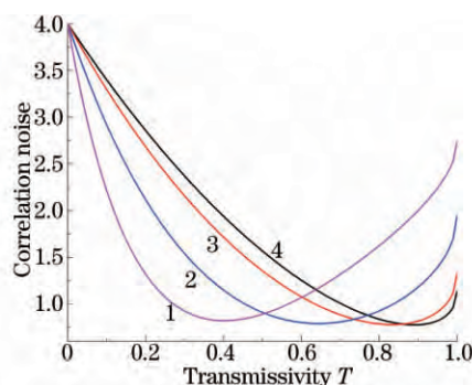
图 3 不同的 \gamma_1 下输出光场关联噪声随 M5 透射率 T 的变化
