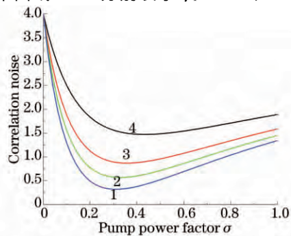
图 4 不同的 \gamma_1 下输出光场关联噪声随抽运功率因子 \sigma 的变化
