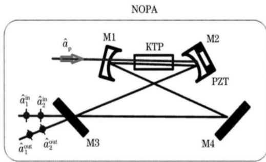
图1 NOPA结构示意图
