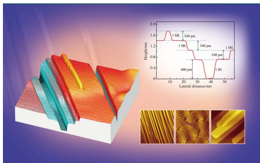
Bi(110)薄膜在NbSe 2 衬底上的扫描隧道显微镜研究 [刘建宇, 孙昊桦, 管丹丹, 李耀义, 王世勇, 刘灿华, 郑浩, 贾金锋 2018 物理学报 67 170701]
