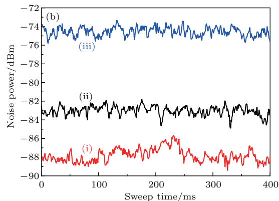
图 5 1.34 \mu\text{m} 真空压缩态光场噪声功率谱 (a) 分析频率为 8 kHz; (b) 分析频率为 36 kHz
