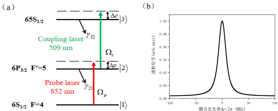
图 1 (a) 铯原子里德伯 EIT 阶梯型能级图； (b) 阶梯型多能级结构理论模拟 EIT 光谱；横坐标为耦合光失谐，纵坐标为 EIT 透射信号强度。
