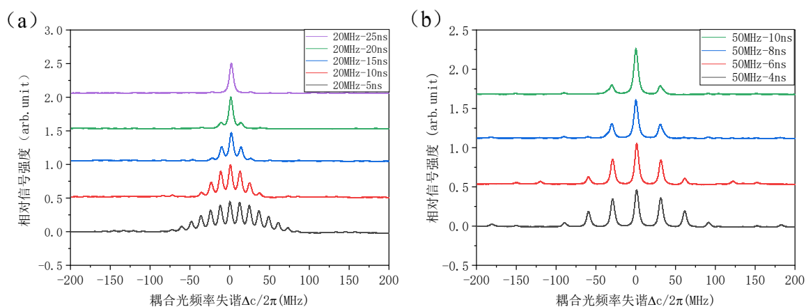
图 6 EIT 信号光谱图 (a) 重复频率为 20 MHz，脉宽分别为 5 ns（灰色）、10 ns（红色）、15 ns（蓝色）、20 ns（绿色）、25 ns（紫色）；(b) 重复频率为 50 MHz，脉宽分别为 4 ns（灰色）、6 ns（红色）、8 ns（蓝色）、10 ns（绿色）
