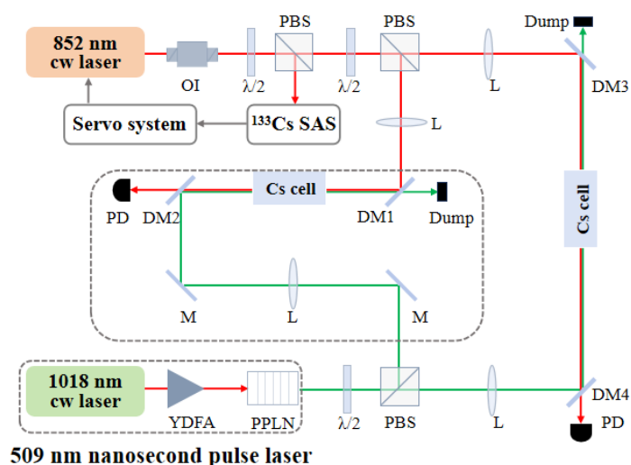
图 3 铯原子光谱实验装置图
