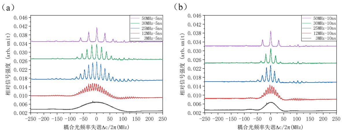
图 5 EIT 信号光谱图 (a) 脉宽为 5 ns，重复频率分别为 3 MHz（黑色）、12 MHz（红色）、25 MHz（蓝色）、30 MHz（绿色）、50 MHz（紫色）； (b)
