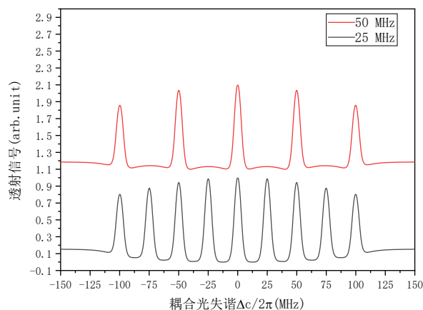
图 2 耦合光为脉冲激光的阶梯型多能级结构理论模拟 EIT 光谱；横坐标为耦合光失谐，纵坐标为归一化的 EIT 透射信号强度。
