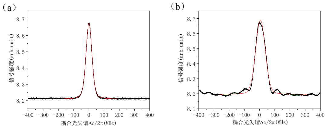
图 4 铯里德伯原子 EIT 光谱 (a) 连续 509 nm 耦合光扫描；(b) 脉冲 509 nm 耦合光扫描
