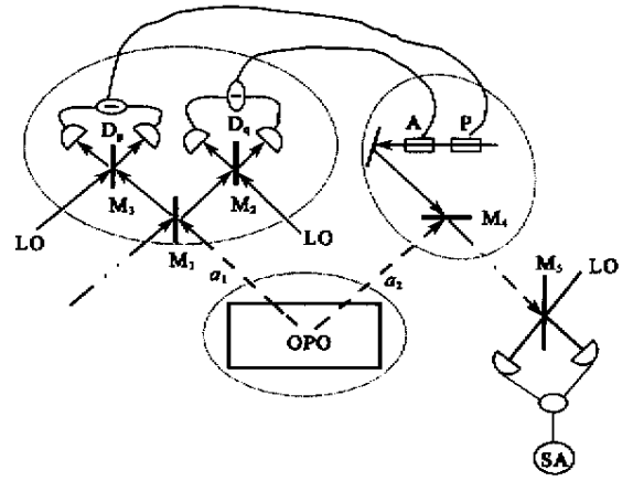
图 1 连续变量量子态的离物传送原理图 (OPO 为光学参量振荡器; a_1 和 a_2 代表 OPO 输出的 EPR 对的两模; M_1, M_2, M_3 为 50% 的分束器; M_4 为反射率很高的分束器; LO 为本底光; SA 为谱分析仪; D_1, D_2 为平衡零拍探测系统; A 为振幅调制器; P 为位相调制器)
