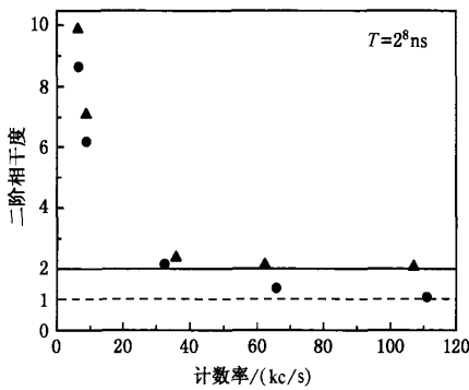
图4 当取样时间 T = 2^8 ns 时,热光场与相干光场的二阶相干度随计数率的变化(图中 \blacktriangle 和 \bullet 分别为热光场与相干光场实验测量结果,实线为热光场理论值,虚线为相干光理论值)
