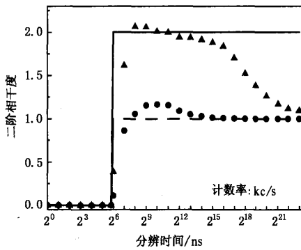
图2 计数率为 109 kc/s 时,热光场与相干光场的二阶相干度随取样时间 T 的变化(图中▲和●分别为热光场与相干光场实验测量结果,实线和虚线分别对应热光场与相干光场的理论分析结果)
