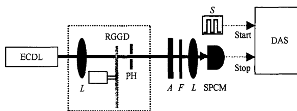
图 1 单探测器直接测量的实验装置图(ECDL 为外腔反馈半导体激光器;L 为凸透镜;RGGD 为旋转的毛玻璃片;PH 为小孔;A 为衰减片;F 为干涉滤光片;S 为信号发生器;SPCM 为单光子探测模块;DAS 为数据采集系统)
