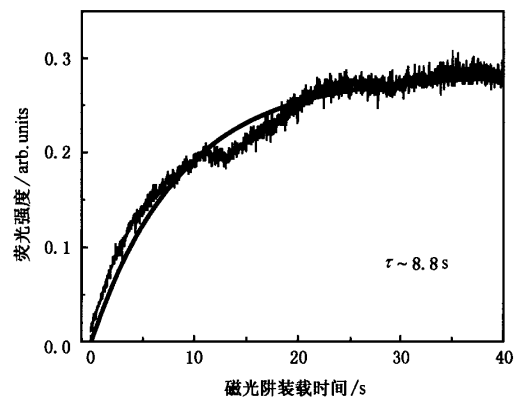
图 4 铯原子磁光阱装载过程中典型的装载曲线. 纵轴的冷原子荧光强度可反映阱中原子数目的相对变化. 拟合得到冷原子在磁光阱中的寿命 \tau \sim 8.8 \text{ s}
