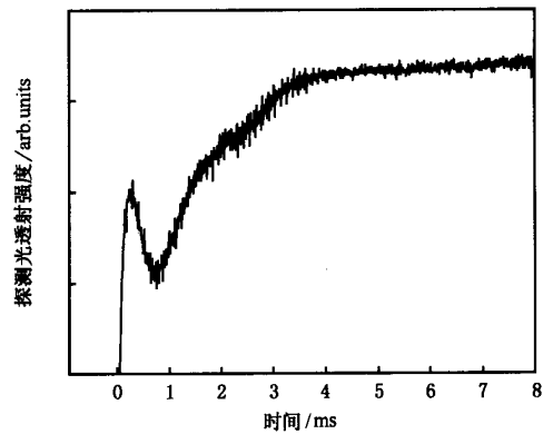
图 2 吸收法测量铯原子磁光阱中俘获的冷原子数目的典型探测光透射信号(向下的凹陷反映原子云对探测光的吸收随着时间的变化)
