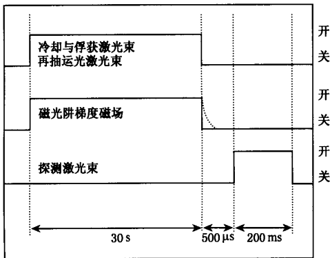
图 1 磁光阱测试系统时序图。磁光阱装载 30s 后,关闭冷却与俘获光和再抽运光激光束(典型关闭时间小于 1 \mu s),同时关闭磁光阱的四极磁场(典型关闭时间小于 450 \mu s),在冷原子云自由膨胀 500 \mu s 后,打开探测激光束测量冷原子对探测光的吸收
