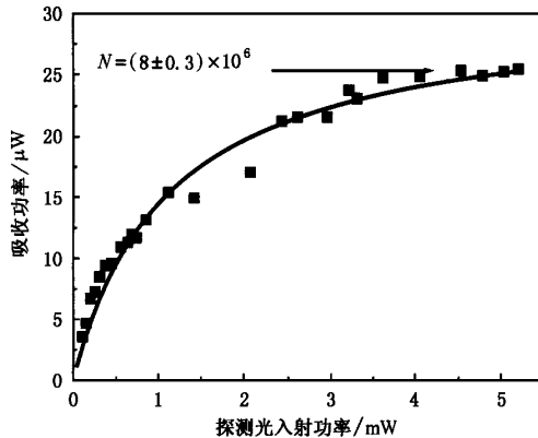
图 3 在不同的探测光功率下测得的冷原子云所吸收的探测光功率(方块是实验测量值, 实线是利用静止二能级原子同共振的单模光场作用的模型拟合得到的结果. 对应的冷原子数目为 (8 \pm 0.3) \times 10^6 )
