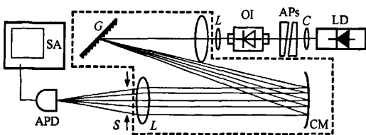
图1 实验装置示意图 C为准直透镜,APs为整形棱镜对,OI为光学隔离器,L为透镜,S为狭缝,G为衍射光栅,CM为凹面镜,APD为雪崩光电探测器,SA为频谱分析仪
