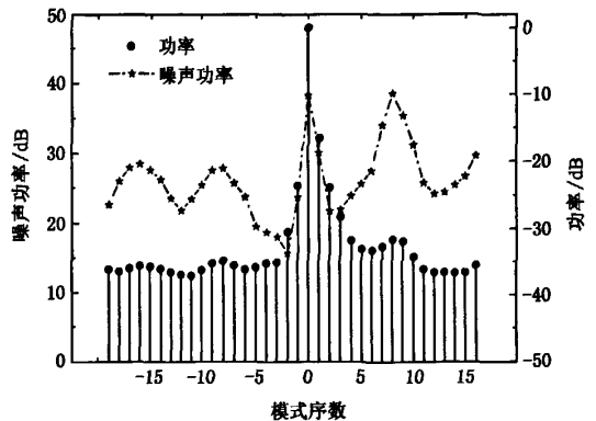
图 4 LD 各纵模的功率与噪声功率随模式数的变化.主模功率取为 0 dB,散粒噪声基准取为 0 dB,LD 的抽运电流为 130 mA
