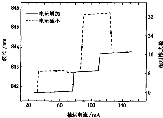
图6 LD的主模波长随抽运电流的变化 LD工作温度为16℃,阈值电流为25 mA.右侧坐标为相对于阈值时LD主模式的纵模数
