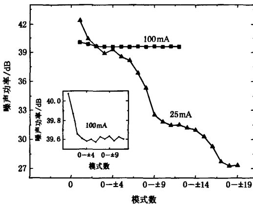
图 3 狭缝以主模为中心向两侧对称打开时,归一化的 LD 强度噪声功率随模式数的变化.散粒噪声基准对应 0 dB.内插图为 100 mA 时的强度噪声功率分布曲线的局部放大
