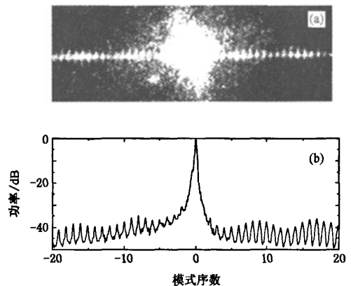
图2 凹面镜焦平面上的纵模功率分布 (a)为CCD拍摄的照片;(b)为扫描狭缝得到的模式功率分布,主模功率为0 dB,横坐标为相对于主模(坐标为0)的模式序号,正方向为波长增大的方向
