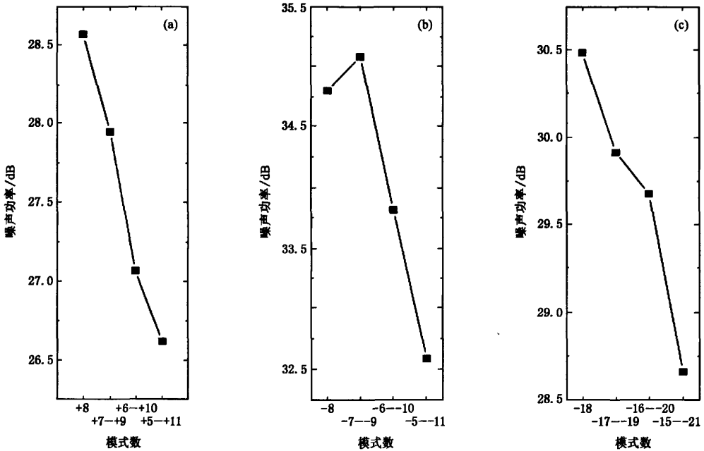
图5 以+8级、-8级、-18级边模为中心对称展开狭缝时,强度噪声功率随模式数的变化 散粒噪声基准对应0 dB。(a)+8级边模,(b)-8级边模,(c)-18级边模
