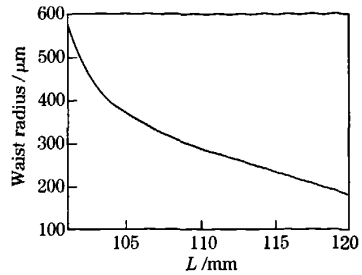
图 2 晶体中振荡激光腰斑半径随凹面镜之间距离的变化关系
