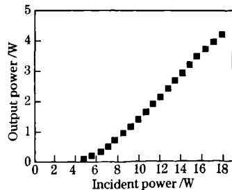
图 3 1053 nm 单频激光输出功率随抽运光功率的变化关系
