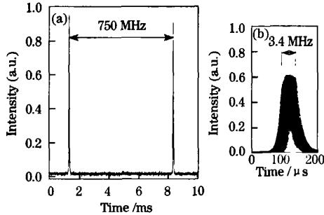
图5 利用扫描共聚焦布里-珀罗腔测量到的激光器单频模式(a)及锁定激光器后激光的频率波动(b)
