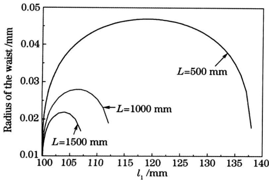
图 3 不同腔长下，振荡光在钛宝石晶体中心处腰斑随两凹面镜之间距离 l_1 的变化关系
