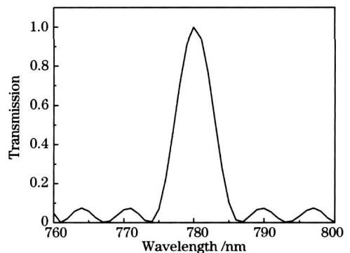
图 5 两片组合双折射滤波片在 760~800 nm 范围内的波长调谐特性曲线
