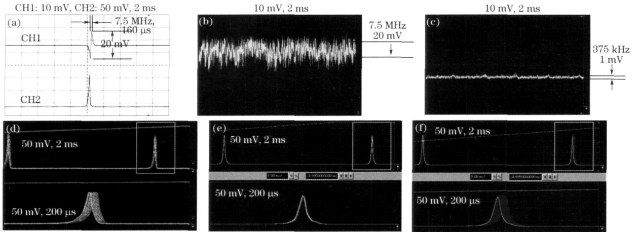
图9 钛宝石激光器的频率稳定性。(a)鉴频曲线;(b)自由运转时激光器的强度波动;(c)激光器锁定后的强度波动;
