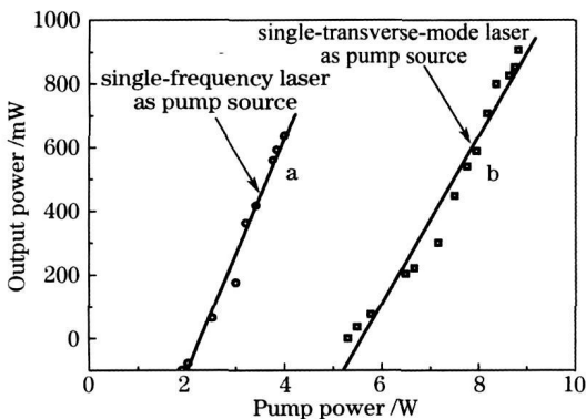
图6 钛宝石激光器的输出功率随抽运功率变化的关系图
