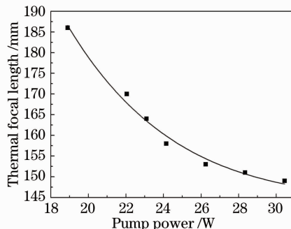
图 6 热透镜焦距随抽运功率的变化
