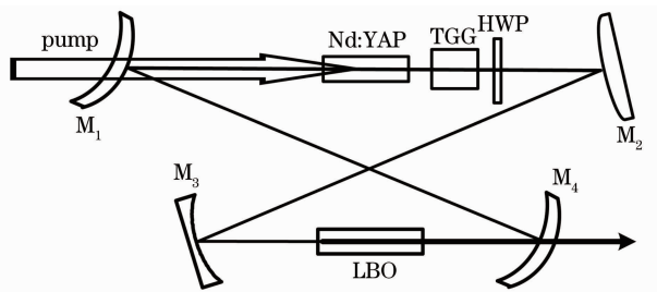
图 4 实验装置图
